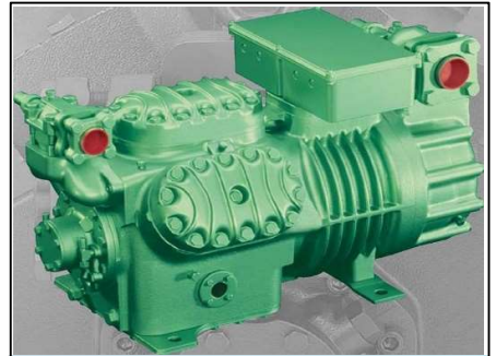
Máy nén Bitzer Piston bán kín
